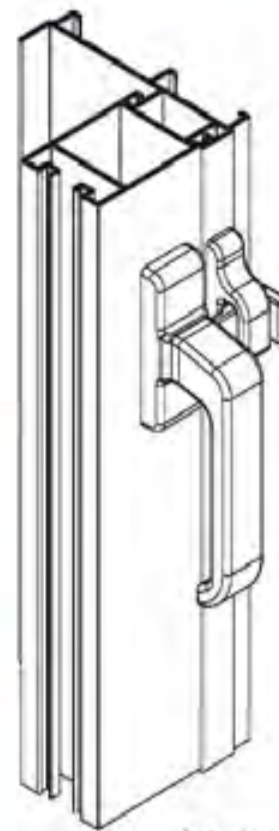
Jaladera Universal Tipo Española para Corrediza ó Proyección Clave-1033-U
