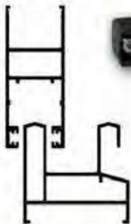
Carretilla Euroalum 4000 Clave-R-40N0
